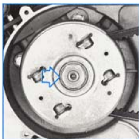
EMBAYAGE
